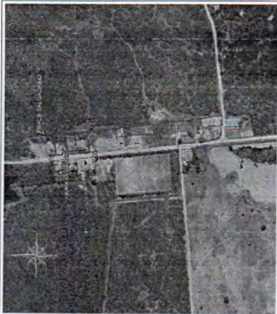
PLANTA DE REFERÊNCIA DA OBRA CORRELAÇÃO COM O PLANO DE COORDENADAS EM UTM - SIRGAS DA UTM-2000
